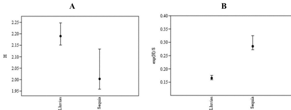
Figura 5. Diversidad (A) y uniformidad (B) de coleópteros asociados a la carroña en la época de lluvias y sequía. Las barras de error corresponden al intervalo de confianza de 95%.
