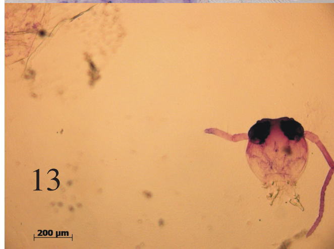
Figuras 9-14. Colémbolos del Nevado de Colima. 9-10. Guthriella muskegis Börner. 9. Macho. 10. Hembra. 11. L. violaceus Fourcroy. 12. Sminthurides macnamarai Folsom & Mills 13. Sminthurus viridis Linnæus. 14. Sphyroteca confusa Snider.
